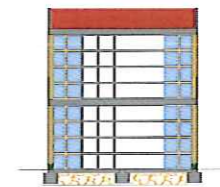
SEZIONE A - A'
